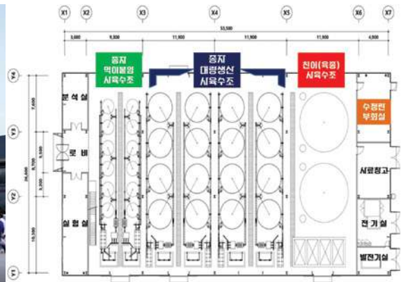
내수면 연어산업화 연구동 배치도
