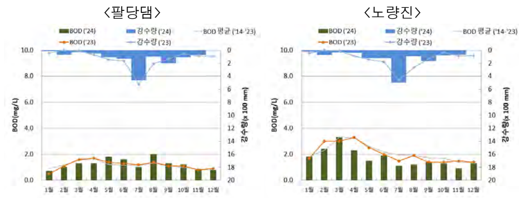
〈그림 2-8-6〉 한강 수계 대표 측정지점 수질변화 추이('24)
