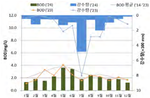
〈그림 2-8-8〉 금강 수계 대표 측정지점 수질변화 추이('24)
