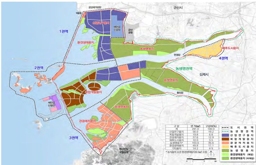
〈그림 2-2-11〉 새만금 권역별 용지계획도
