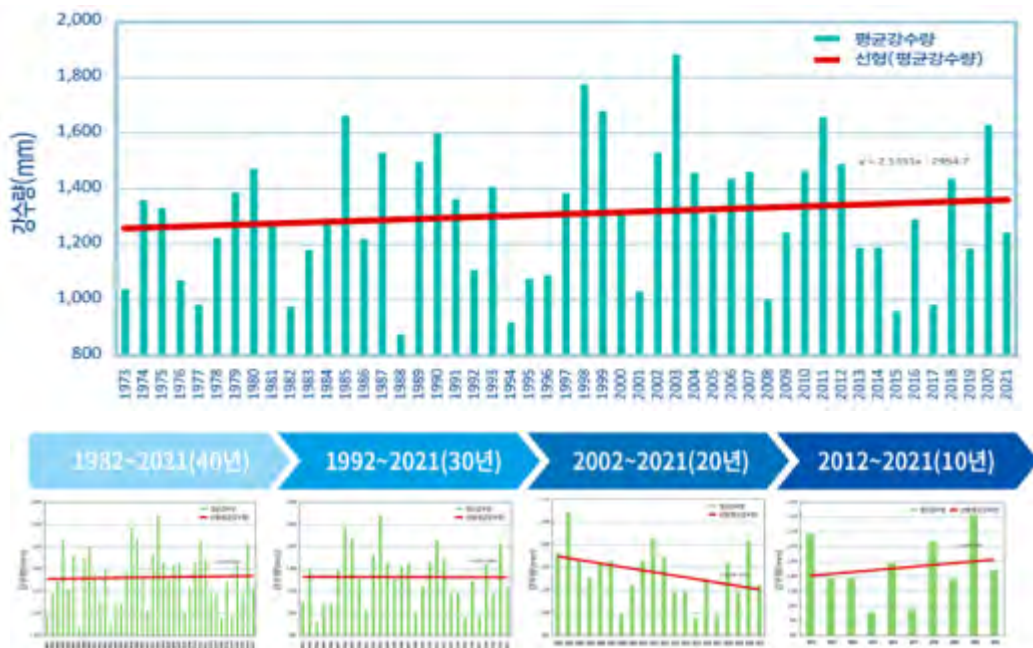
〈그림 2-7-1〉 전국 연평균 강수량 변화
