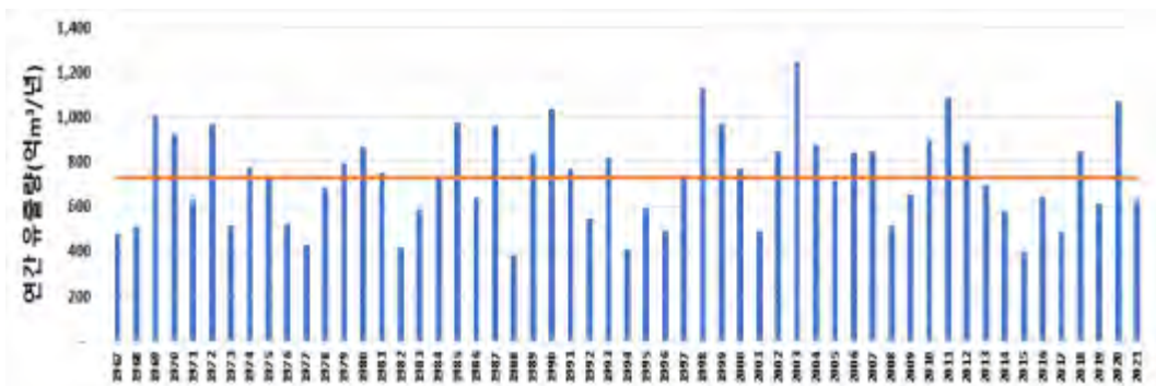
〈그림 2-7-2〉 우리나라 연평균 유출량 추이(1967~2021년)
