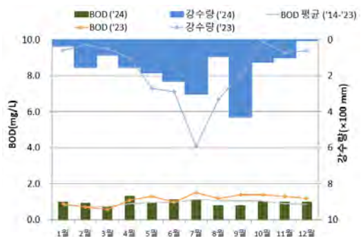
〈그림 2-8-9〉 영산강·섬진강 수계 대표 측정지점 수질변화 추이('24)
