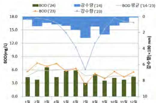
〈그림 2-8-9〉 영산강·섬진강 수계 대표 측정지점 수질변화 추이('24)
