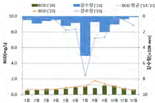
〈그림 2-8-8〉 금강 수계 대표 측정지점 수질변화 추이('24)
