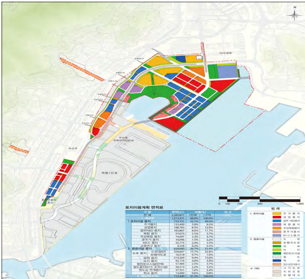
〈그림 2-6-19〉 부산북항 2단계 토지이용계획(부산시컨소시엄(안, '20.5.)
