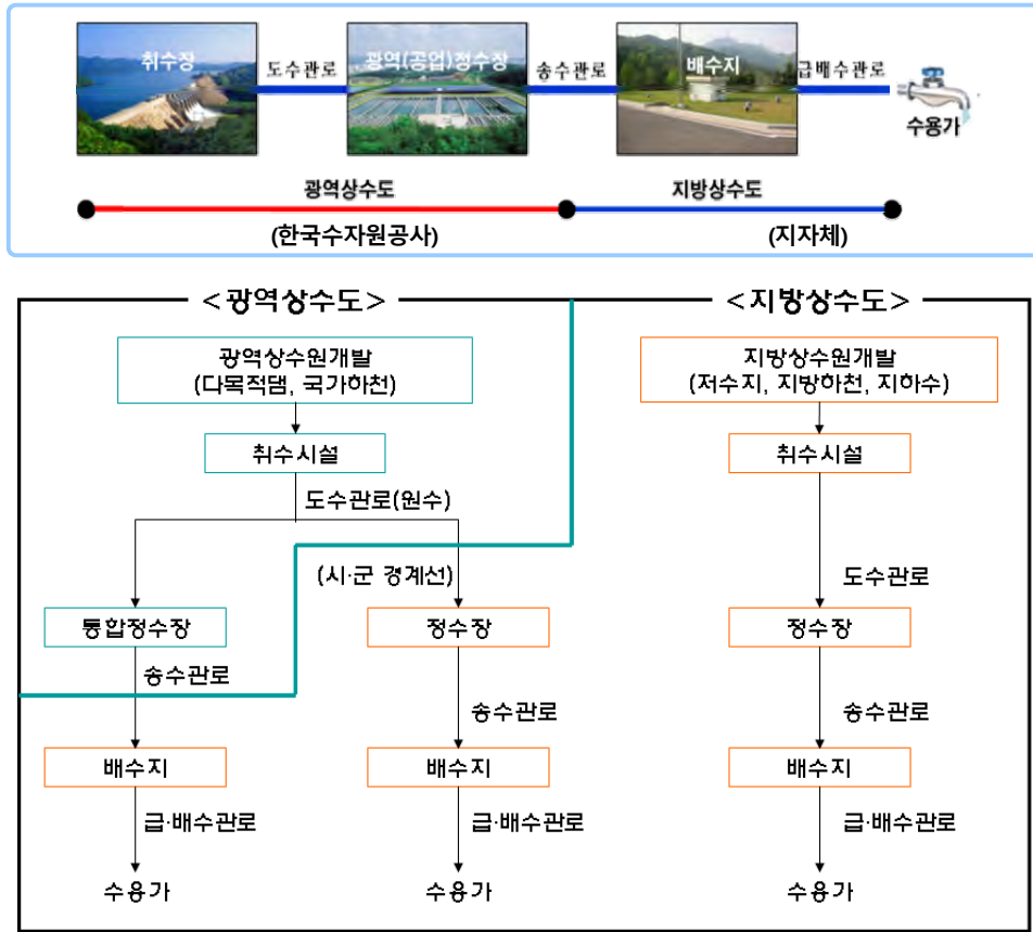
〈그림 2-7-13〉 상수도 관리체계 모식도
